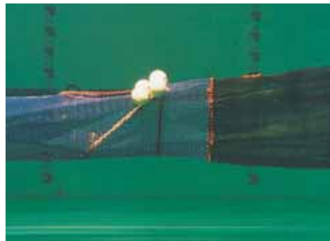
Este TED es usado en pesquerías estuarinas de Este australiano. El ángulo de la parrilla es de 45°.
