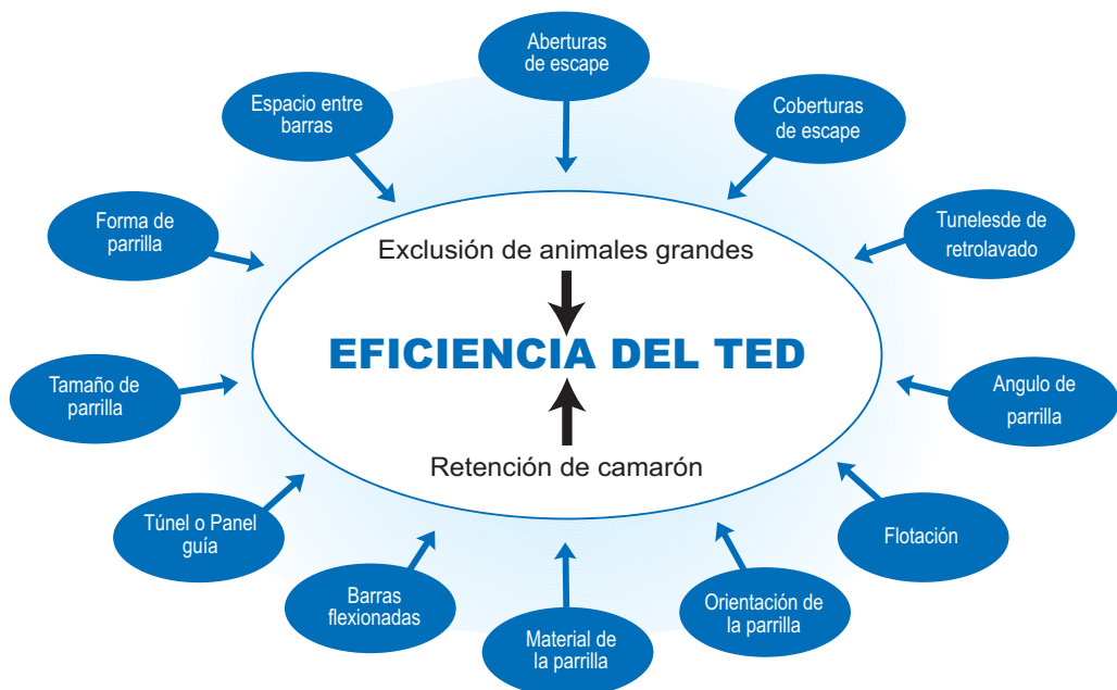
Los diferentes diseño y parámetros de construcción que influyen en la eficiencia y funcionamiento del TED. Observe que una falla excluyendo animales grandes esta ligada como una causa de pérdida de camarón.
