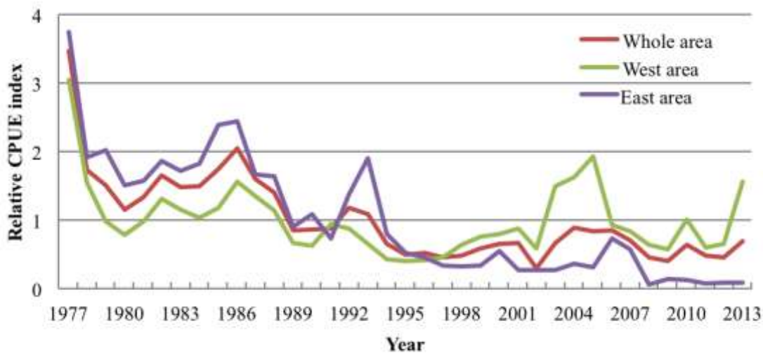
Figure 17. Albacore : comparaison des séries de PUE palangrières normalisées de Rép. de Corée. Les séries ont été ajustées à leur moyenne respective entre 1977 et 2013.
