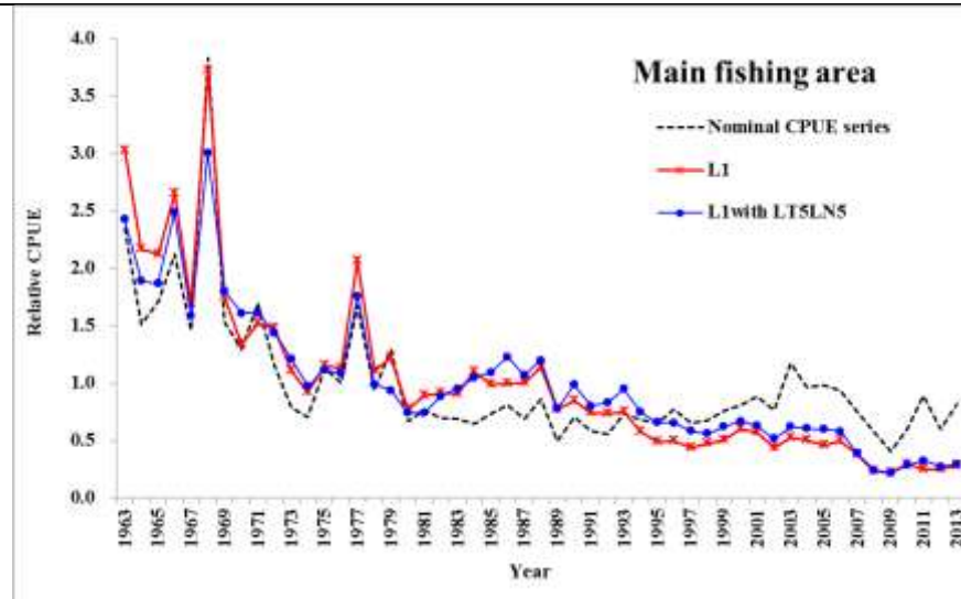
Figure 16. Albacore : Comparaison des PUE annuelles agrégées par zones entre les modèles, avec l'effet des sous-zones et de LT5LN5, normalisées pour les principales zones de pêche, exprimées sur une échelle relative, avec les PUE nominales superposées. Les séries ont été ajustées à leur moyenne respective entre 1963 et 2013.
