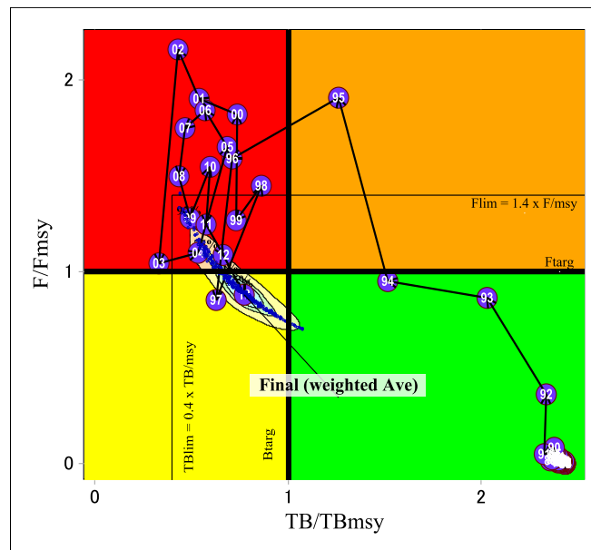
Figure 2. Espadon : Graphe de Kobe pour l'évaluations ASPIC dans le sud-ouest de l'océan Indien (la ligne bleue horizontale représente F_{LIM} , la ligne bleue verticale représente B_{LIM} ). Les résultats correspondent à la meilleure option du modèle : moyenne pondérée du modèle utilisant l'inverse de l'erreur quadratique moyenne des scénarios 2 et 4 (IOTC–2014–WPB12–24 Rev_2).
