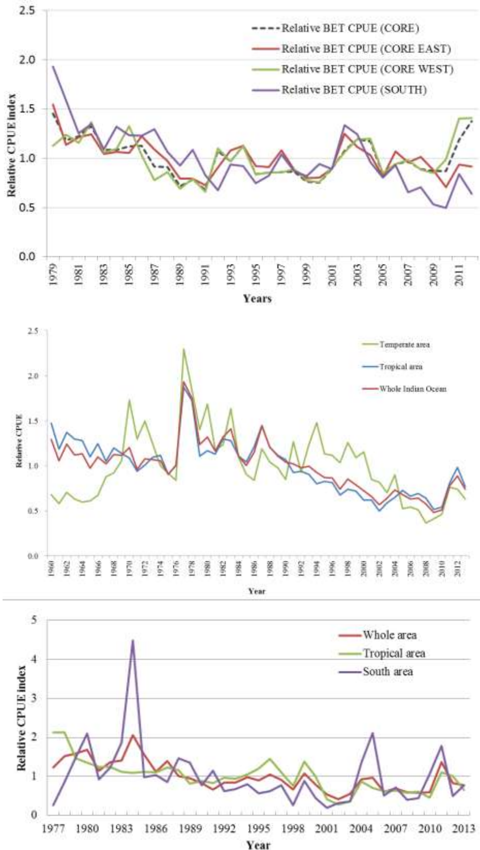
Figure. 14. Patudo : séries de PUE normalisées. haut) comparaison des séries de PUE palangrières normalisées (par zones) de Taïwan, Chine. Les séries ont été ajustées à leur moyenne respective entre 1979 et 2012 ; milieu) comparaison des séries de PUE palangrières normalisées du Japon. Les séries ont été ajustées à leur moyenne respective entre 1960 et 2013 ; bas) comparaison des séries de PUE palangrières normalisées de la Rép. de Corée. Les séries ont été ajustées à leur moyenne respective entre 1977 et 2013.
