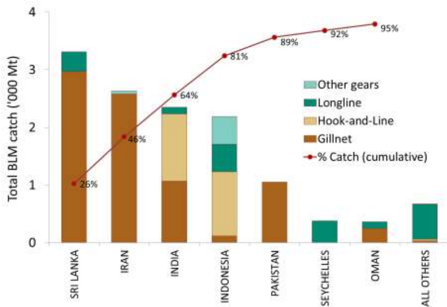
Figure 4. Marlin noir : captures moyennes dans l'océan Indien entre 2010 et 2013, par pays. Les pays sont classés de gauche à droite par ordre de captures de marlin noir décroissantes. La ligne rouge représente le pourcentage cumulé des captures de marlin noir pour les pays concernés par rapport au total des captures combinées de cette espèce pour tous les pays et toutes les pêcheries.
