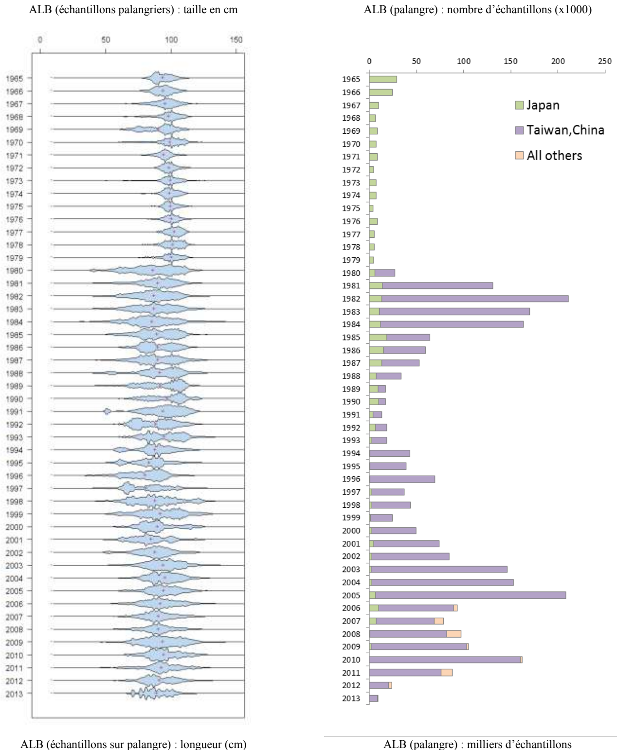
Figure 8a-b. Germon : Gauche : distributions des fréquences de tailles (nombre total de poissons mesurés par classes de tailles de 1 cm) dérivées des données disponibles au Secrétariat de la CTOI pour les palangriers surgélateurs, par années. Droite : Nombre de spécimens échantillonnés pour la longueur par les principales flottilles de palangriers.
