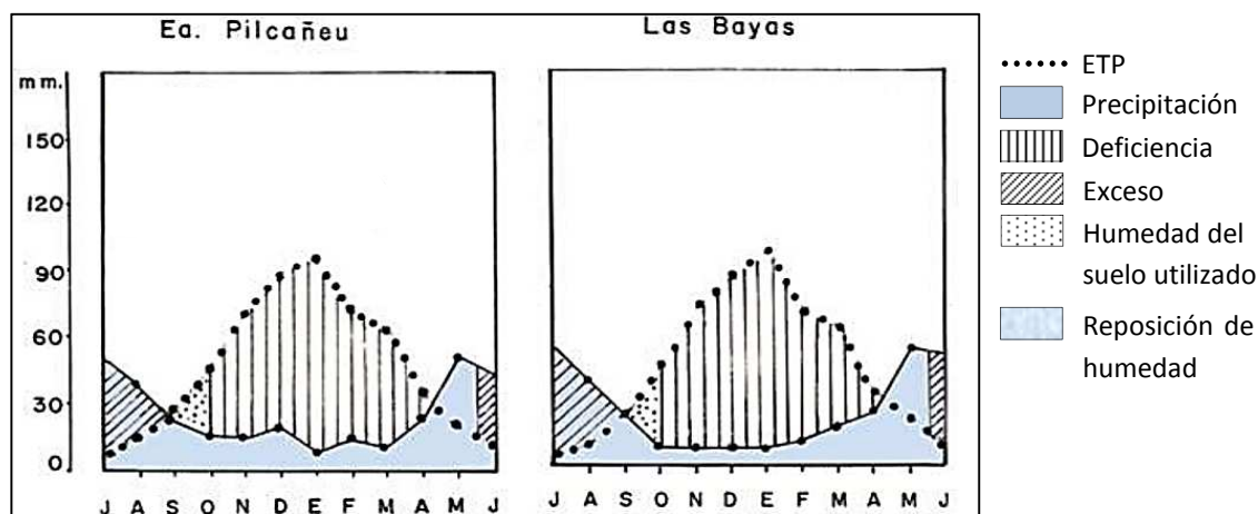
FIGURA 9 - BALANCE HÍDRICO EA. PILCAÑEU Y LAS BAYAS
