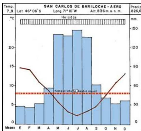
FIGURA 10 - CLIMATOGRAMA DE SAN CARLOS DE BARILOCHE. PERÍODO 1941-80 - SMN
