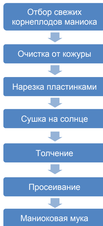
Рис. 4. Технологическая схема производства неферментированной маниоковой муки.
