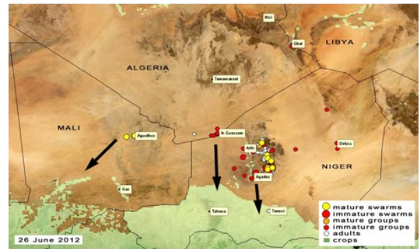
Figure 2 : Situation acridienne au 26 juin 2012
