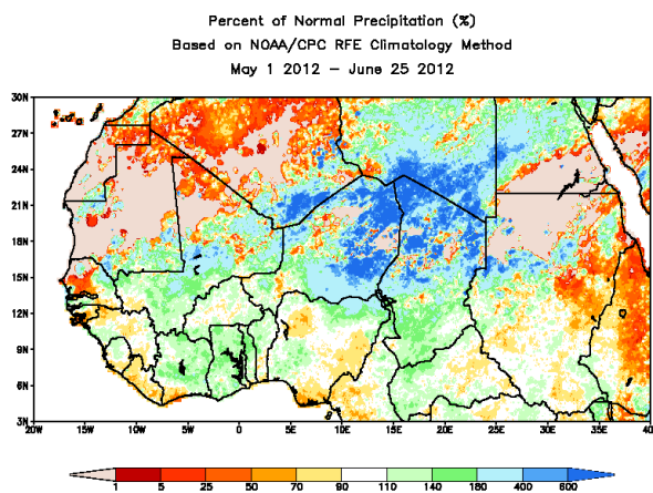
Figure 1 : Anomalie de pluviométrie (en pourcentage par rapport à la moyenne 1983-2011)
