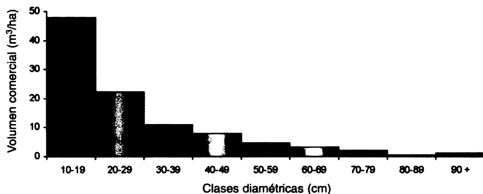
Figura 4.6 Distribución del volumen comercial (m³/ha) por clase diamétrica en un bosque primario de La Mosquitia de Nicaragua
