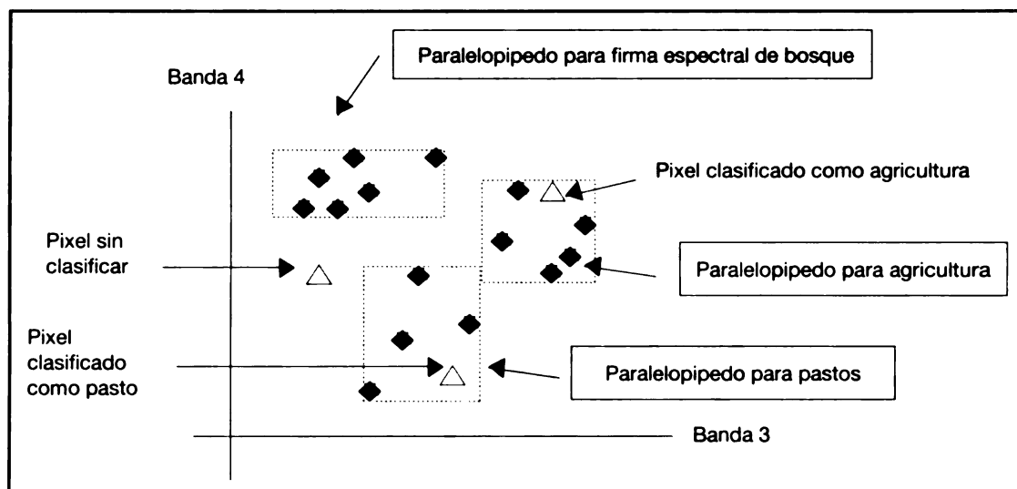
Figura 3.6 Esquema del funcionamiento del método de clasificación de paralelepípedos
