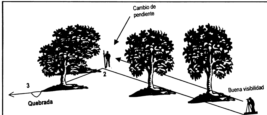
Figura 3.9 Levantamiento con brújula y cinta: se miden tramos con buena visibilidad y pendientes constantes
