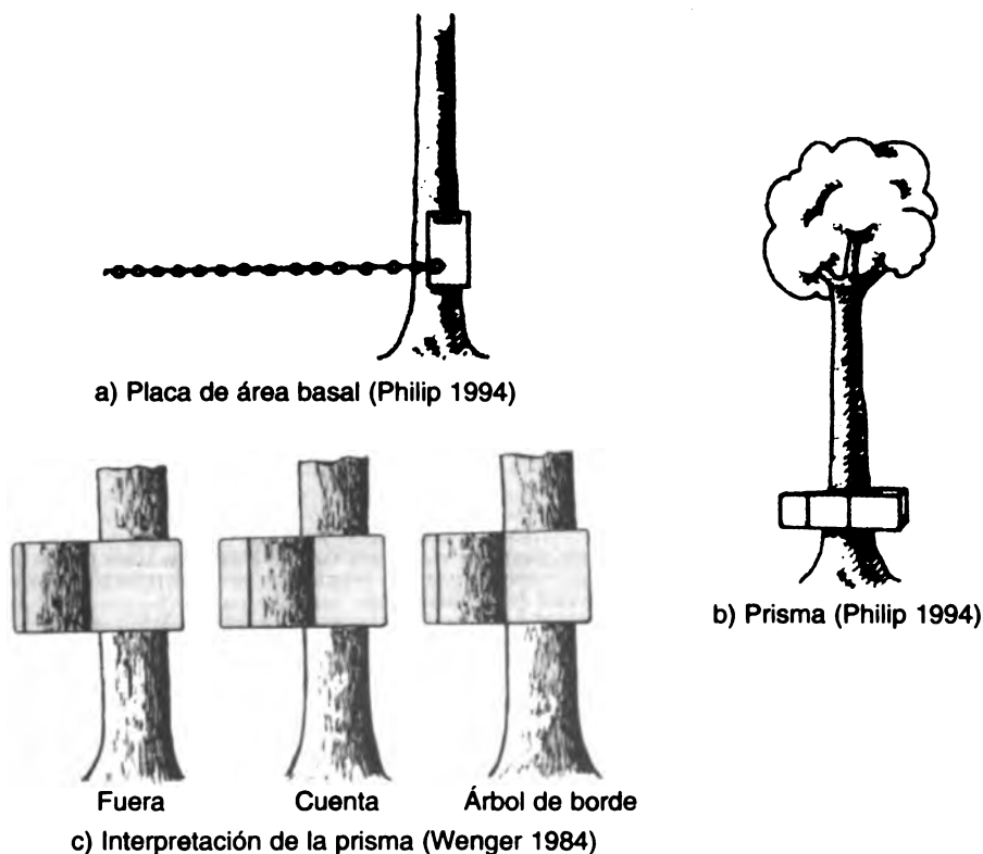
Figura 7.2 Instrumentos usados para el muestreo de áreas variables Fuentes: Wenger (1984), Philip (1994)
