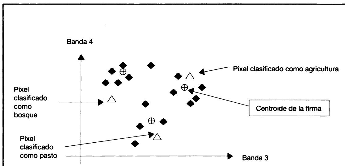
Figura 3.7 Esquema de funcionamiento del método de clasificación de distancia mínima
