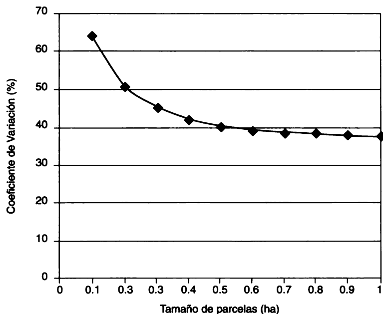
Figura 5.2 Curva área-coeficiente de variación respecto del volumen comercial de todas las especies (dap >25 cm) para el bosque primario en Arroyo Colorado, Petén, Guatemala. Fuente: Carrera (1996)
