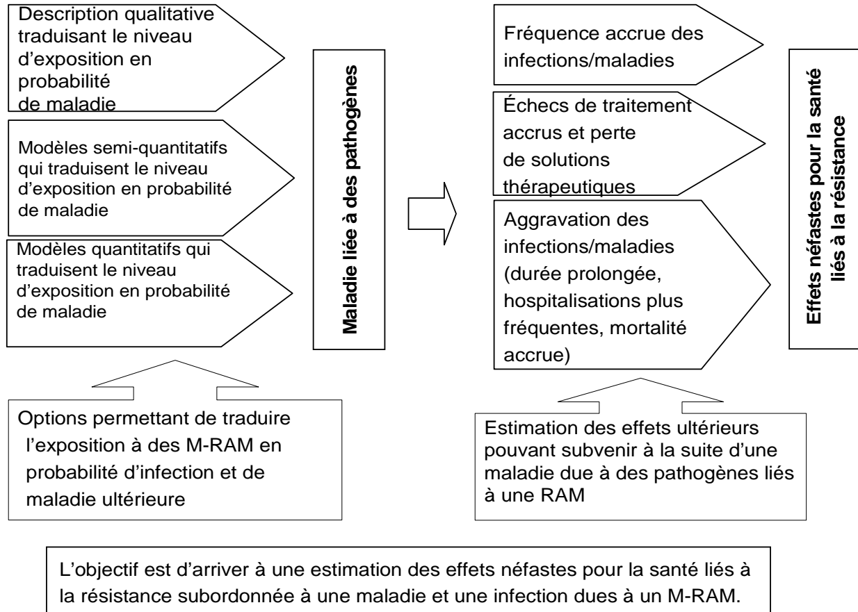
Figure 2b. Éléments à prendre en compte pour la caractérisation des dangers dans une évaluation des risques liés à la RAM d'origine alimentaire
