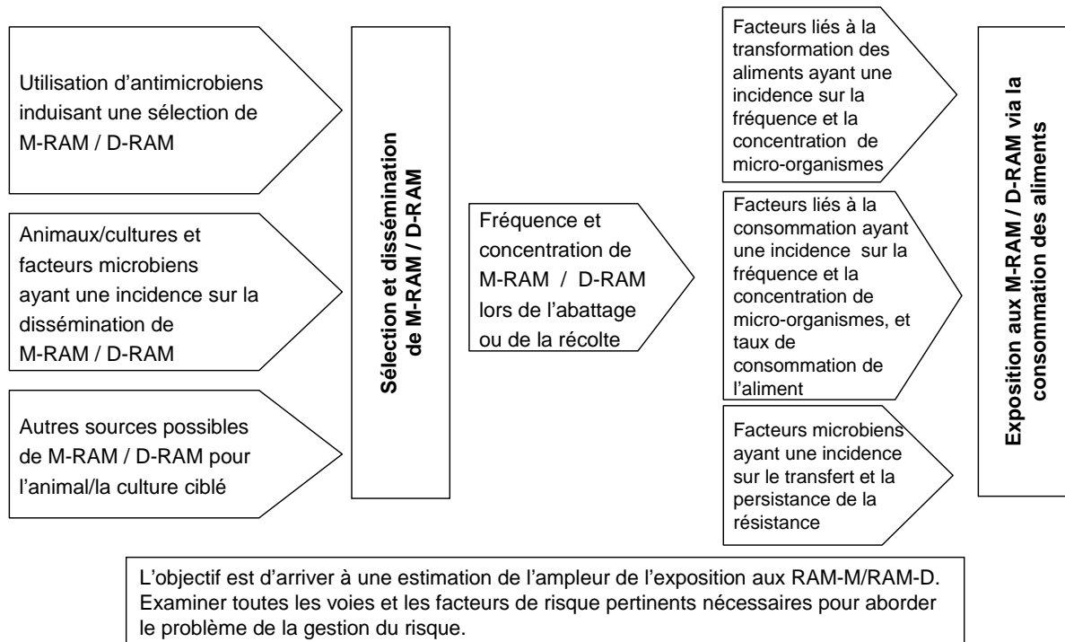
Figure 2a. Éléments à prendre en compte pour l'évaluation de l'exposition dans les évaluations des risques liés à la RAM d'origine alimentaire – la voie d'exposition
