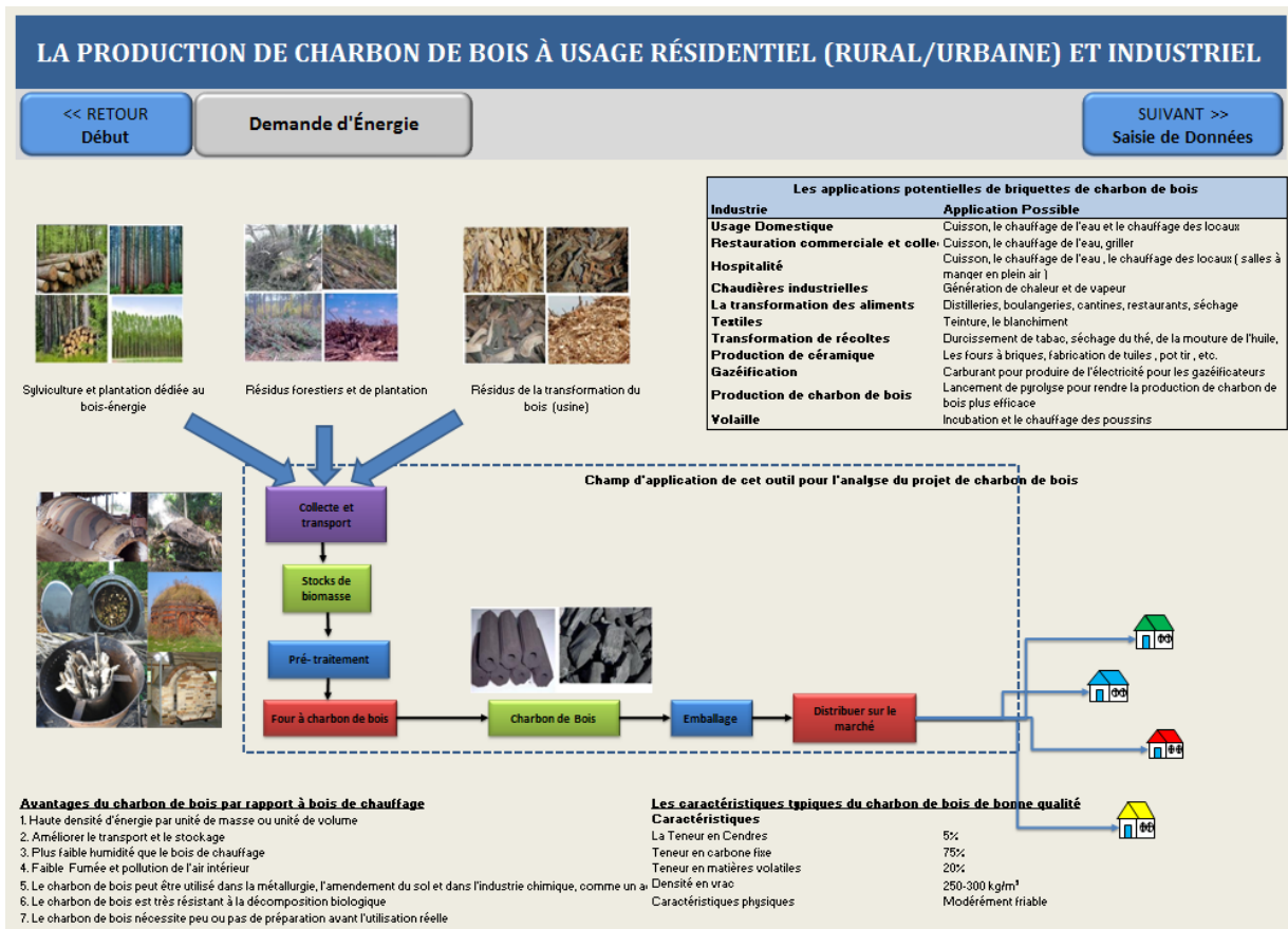
Figure 2: Système de Charbon de Bois pour le Chauffage et la Cuisson dans les Zones Rurales et Urbaines
