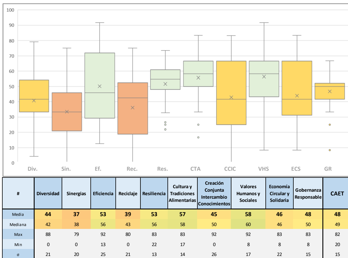
Figura 10: Caracterización de la transición agroecológica (CAET) para toda la muestra en el AMR: Resultados desagregados para los 10 Elementos de la Agroecología.
