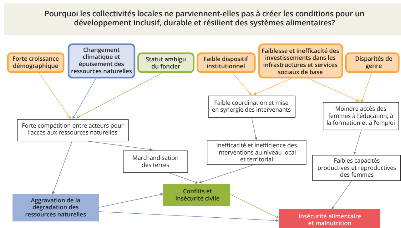
Figure 24. Représentation systémique de la QCD 3
