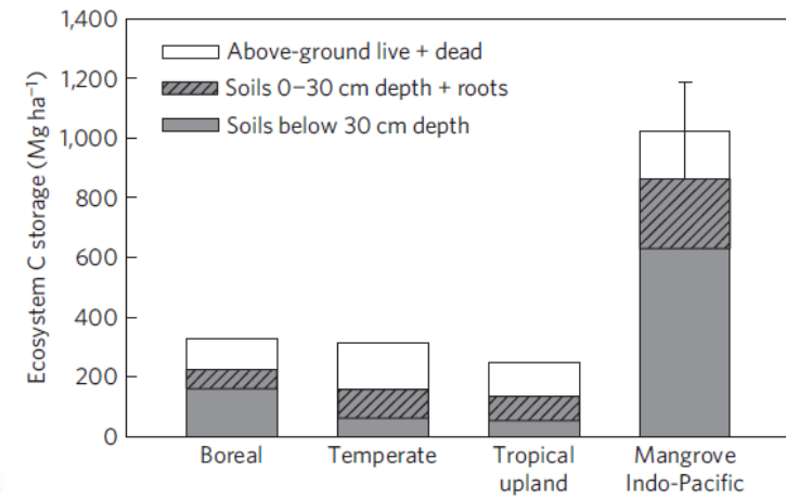
Donato et al. Nature Geosci (2011)
