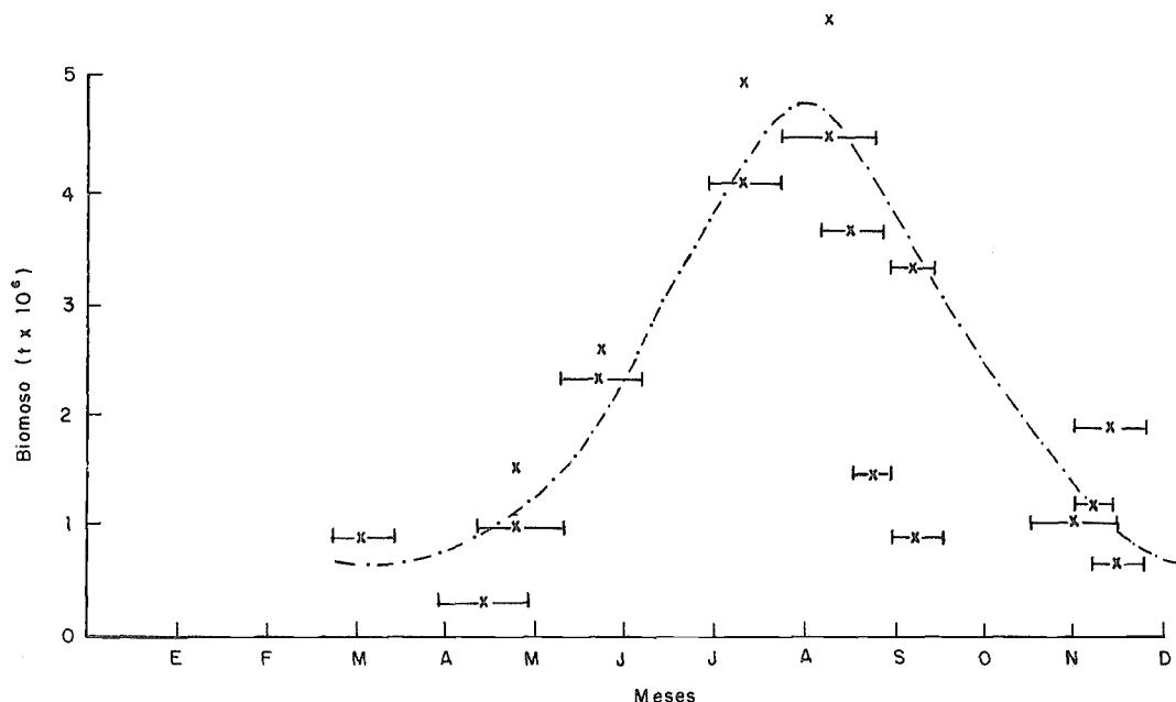
Fig.18 Biomasa de sardina española estimadas con métodos hidro-acústicos entre Arica y Antofagasta (0-200 millas n.) en 1981-1985 (del Instituto de Formento Pesquero, 1985)
