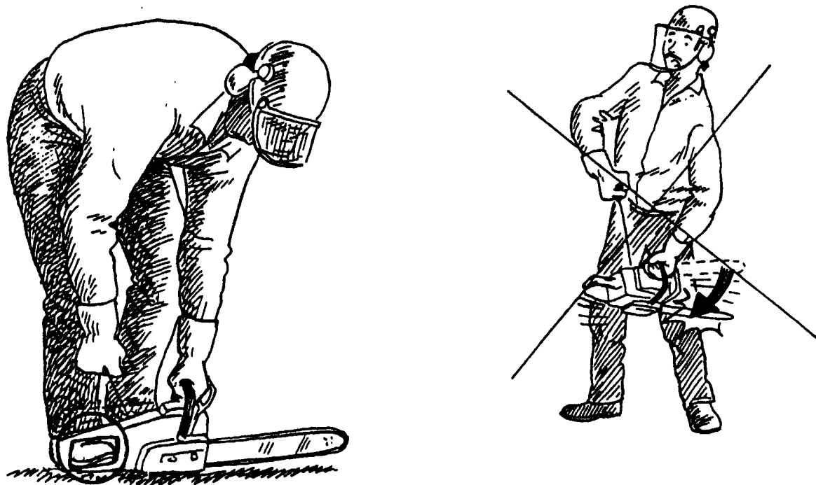
Figura 40a. Como encender la motosierra en el suelo.
