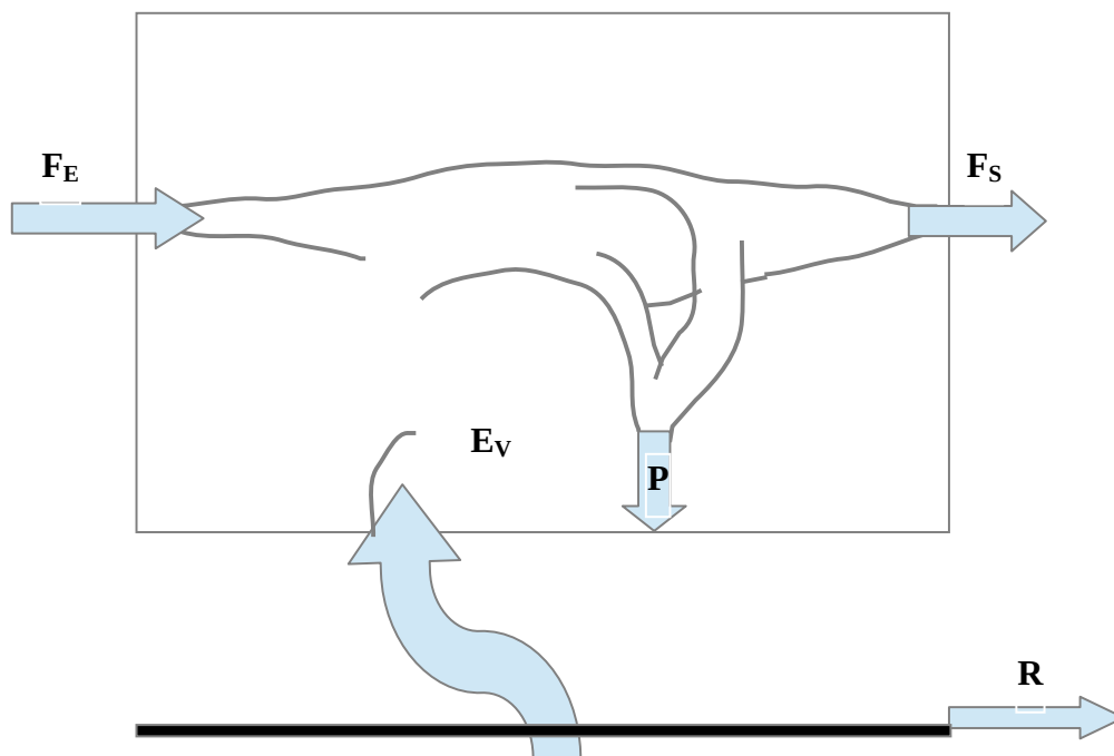
Figure 1 : Modèle conceptuel du cycle de l'eau à travers une région continentale. Le terme F_E représente le flux de vapeur d'eau entrant, F_S le flux de vapeur d'eau sortant, E_v l'évapotranspiration, P la précipitation et R les ruissèlements. L'évaporation des surfaces humides et la transpiration des plantes approvisionnent l'atmosphère en vapeur d'eau, dont une partie retombe sous forme de précipitation et l'autre transporté hors de la région.
