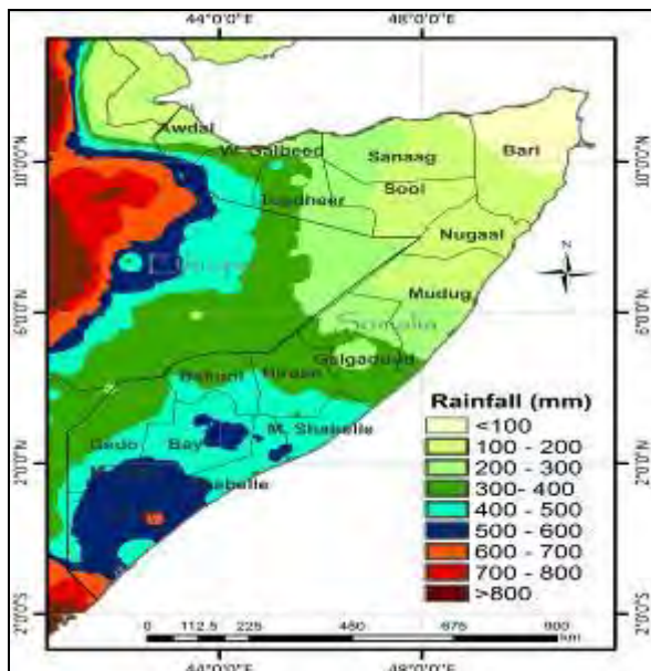
Figure 1: Distribution spatiale des précipitations annuelles moyennes
