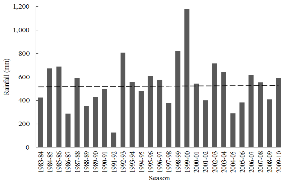
Figure 1: Précipitations saisonnières du Parc National du Gonarezhou, au Zimbabwe entre 1983 et 2010. La ligne en pointillé représente la moyenne à long terme
