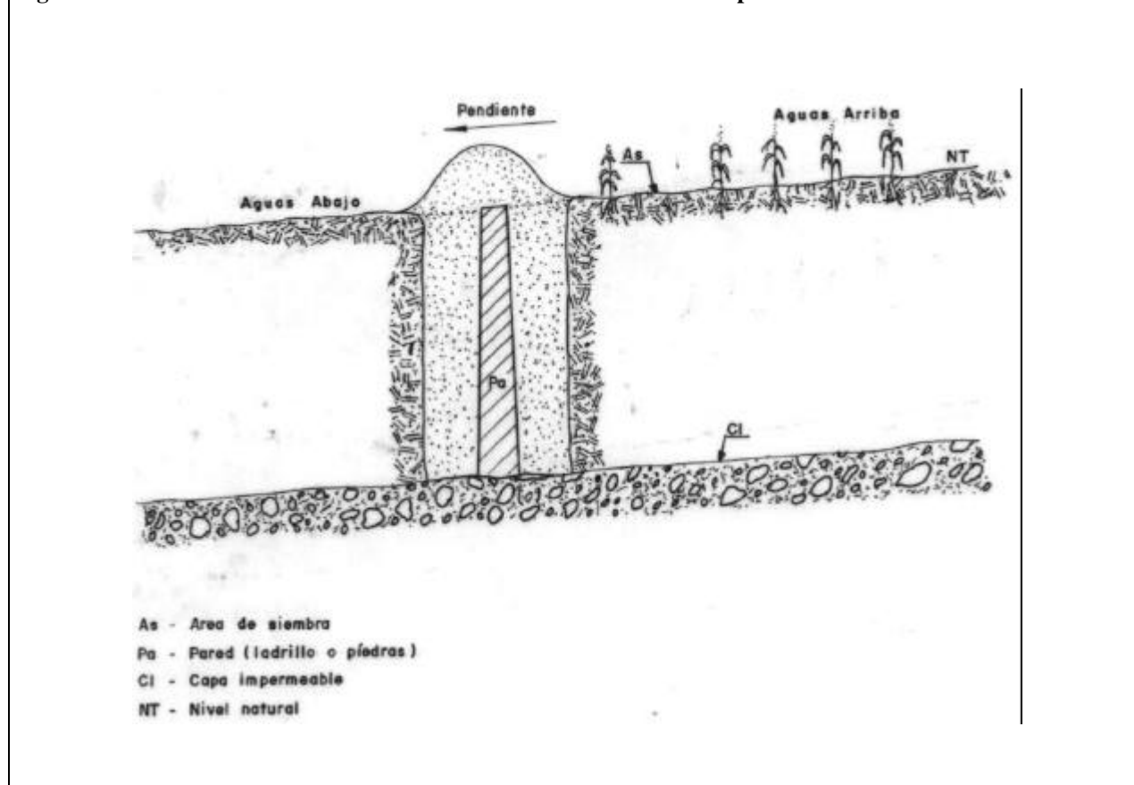
Figura 54. Pared del embalse subterráneo construido con ladrillos o piedras.
