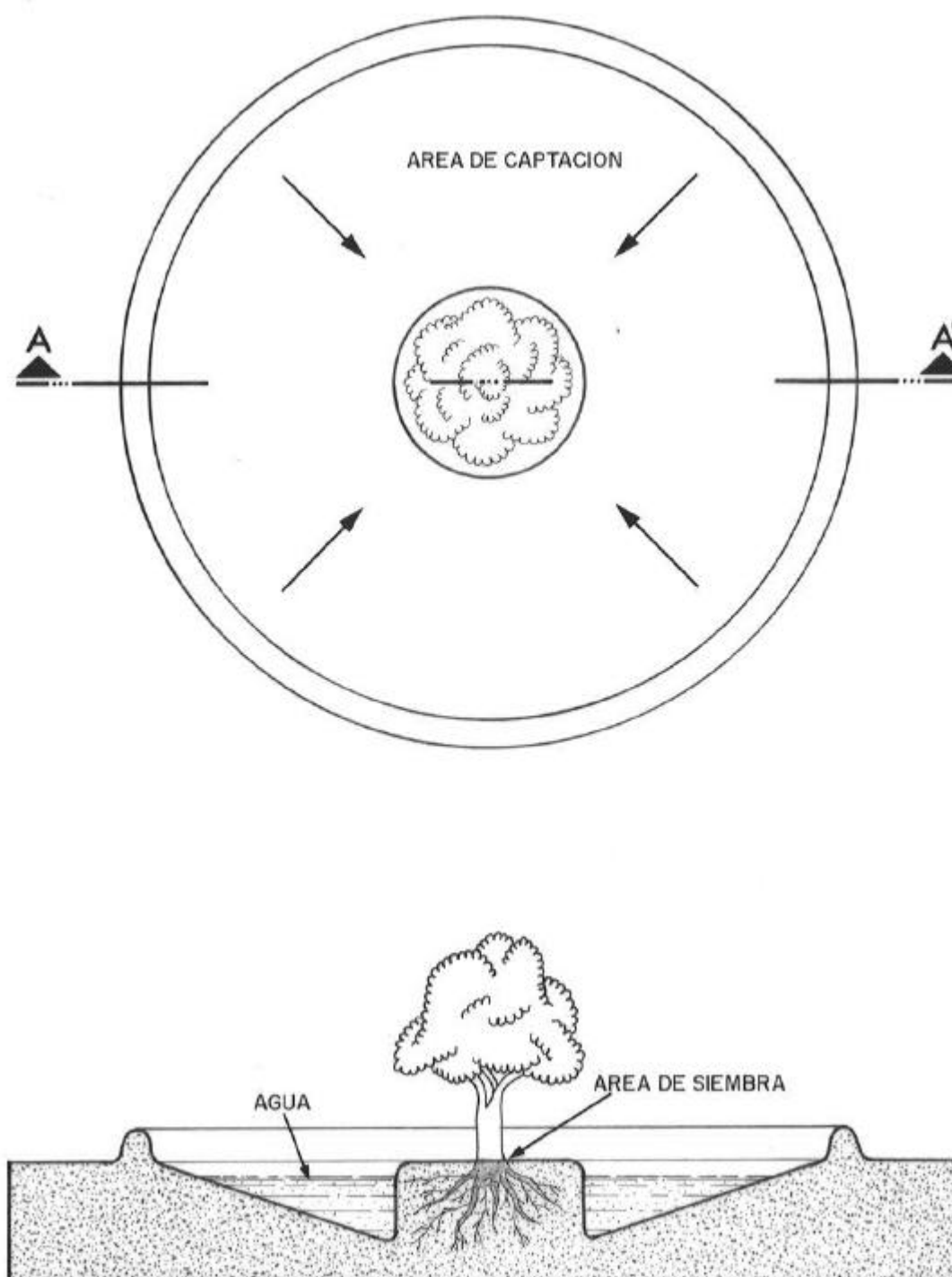
Figura 22. Modelo esquemático de la técnica de captación de agua de lluvia in situ para frutales o cultivos perennes con microcuencas de captación individual para cada árbol.
