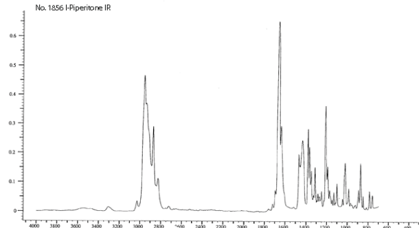
1856 1-Piperitone (MS)
