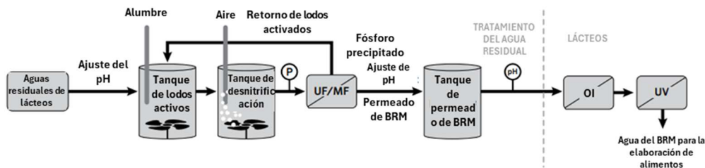
Figura 47: Ejemplo de recuperación de agua de efluentes lácteos mediante un biorreactor de membrana y OI.
