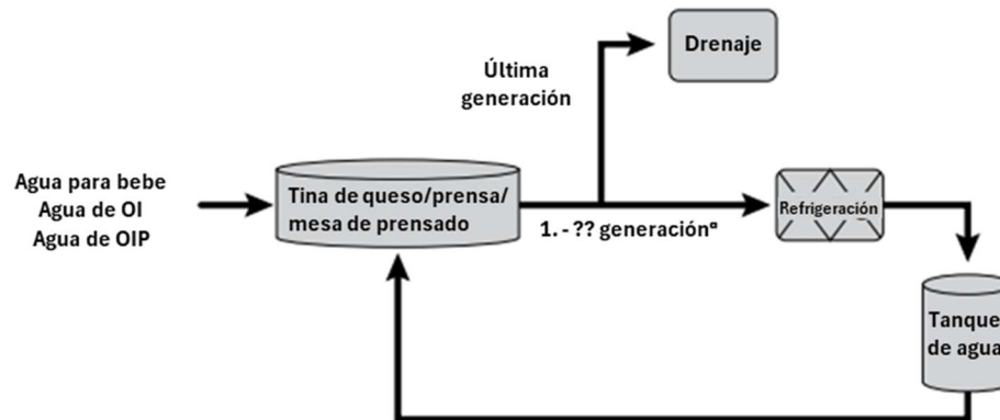
Figura 14: Esquema de la recirculación del agua utilizada para enfriar quesos.
