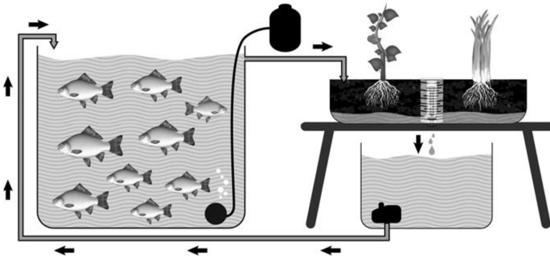
Figura 41: Esquema de una unidad acuapónica simple 4
