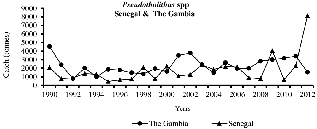
Figure 3.9.3a: Pseudolithus spp. Total landings by country in the CECAF northern sub-area Pseudolithus spp. Débarquements totaux, par pays, dans la sous-région Nord du COPACE
