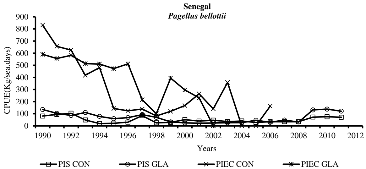
Figure 3.3.3c: Catch per unit effort (CPUE) of the main fleets fishing Pagellus bellottii in Senegal Capture par unité d'effort (CPUE) des principales flottilles pêchant Pagellus bellottii au Sénégal
