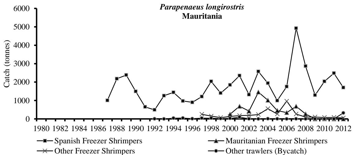
Figure 4.3.3b: Catches (tonnes) by country of deep water pink shrimp ( Parapenaeus longirostris ) of the main fleets fishing in the CECAF northern subregion Captures (tonnes) par pays de la crevette rose en eau profonde ( Parapenaeus longirostris ) des principales flottilles penchant dans la sous-région nord du COPACE
