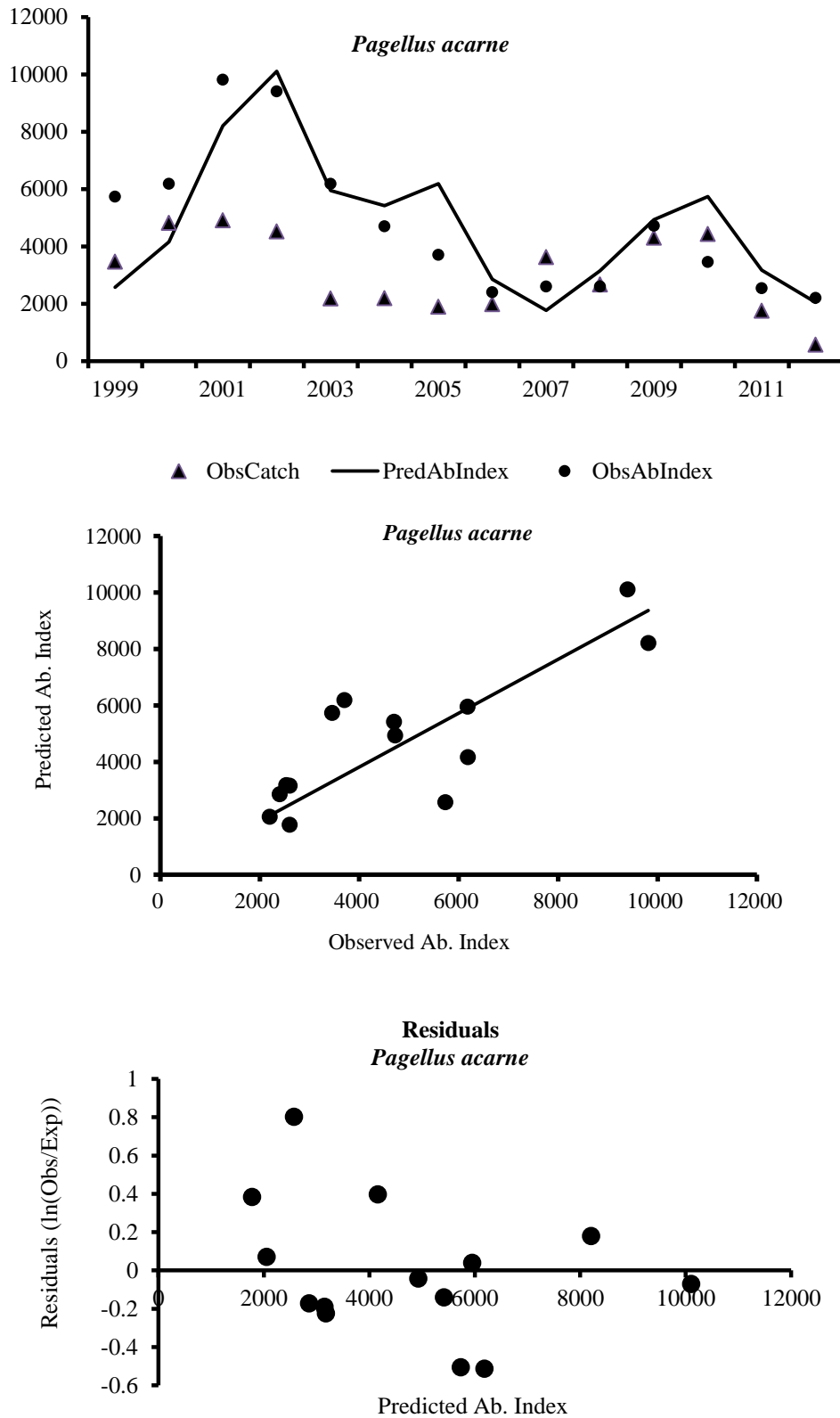
Figure 3.4.4: Pagellus acarne . Trends in the observed and estimated abundance indices and diagnostics of the model fit Tendances des indices d'abondance observés et estimés ainsi que des diagnostics du modèle
