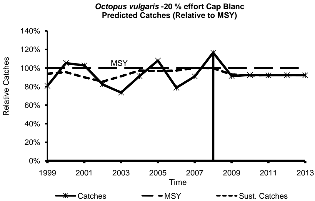
Figure 5.3.5d : Predicted catches and abundance of Octopus vulgaris Cap Blanc stock – Scenario2 (-20% effort) Prédications des captures et de l’abondance de Octopus vulgaris stock de Cap Blanc– Scénario 2 (-20% effort)
