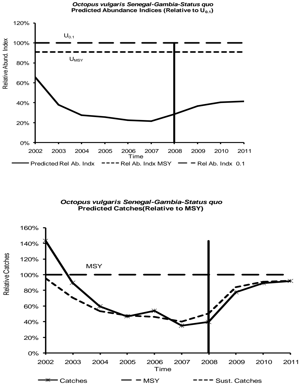
Figure 5.3.5e: Predicted catches and abundance of Octopus vulgaris Senegal-Gambia stock – Scenario1 ( Status quo ) Prédiction des captures et de l'abondance de Octopus vulgaris stock de Cap Blanc– Scénario 1 ( Status quo )
