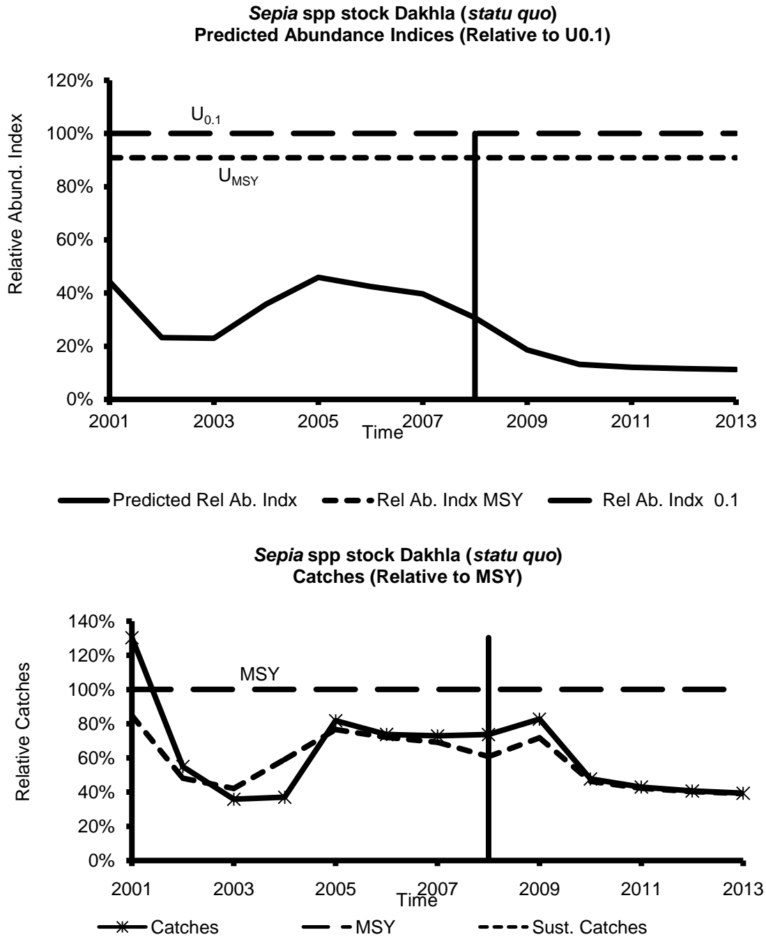
Figure 5.4.5a: Predicted catches and abundance of Sepia spp. Dakhla stock – Scenario 1 ( status quo ) Prédictions des captures et de l'abondance de Sepia spp. stock de Dakhla– Scénario 1 ( status quo )
