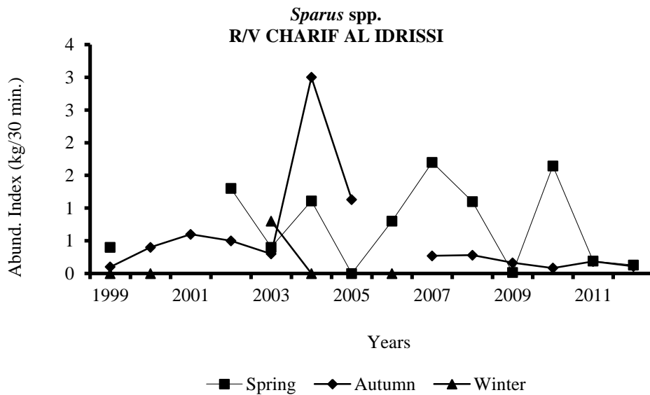
Figure 3.7.3c: Sparus spp. Abundance indices (kg/30 min) obtained during the scientific surveys in Morocco with R/V CHARIF AL IDRISSEI Sparus spp. Indices d'abondance (kg/30 min) obtenus lors des campagnes scientifiques au Maroc avec le N/R CHARIF AL IDRISSEI
