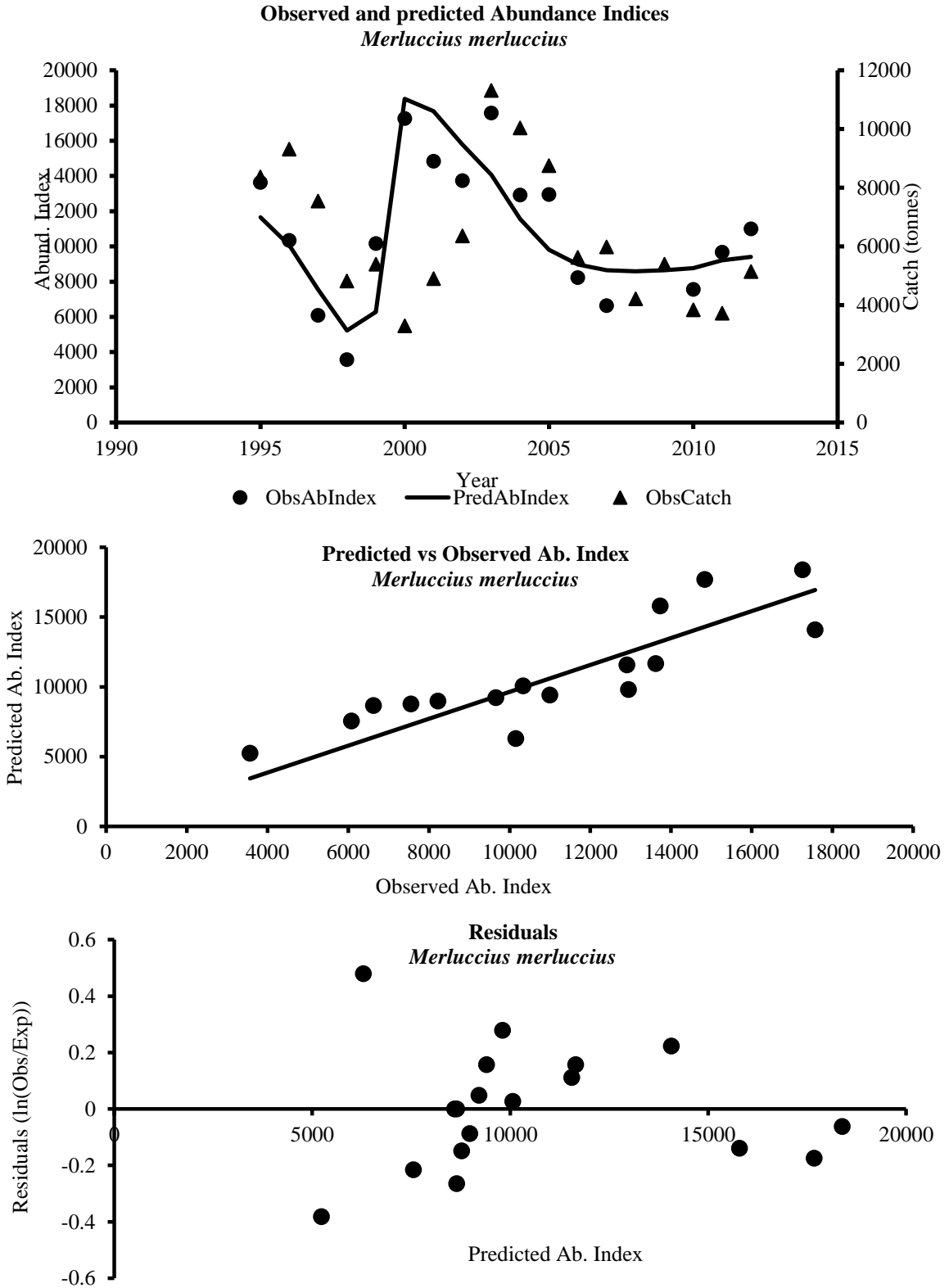
Figure 2.3.4a: Observed and predicted abundance indices for the white hake ( Merluccius merluccius ) stock (abundance indices-survey), and diagnostics of the model fit Tendances des indices d'abondance observés et estimés par le modèle de production pour le stock de merlu blanc ( Merluccius merluccius ) (indices d'abondance-campagnes) ainsi que des diagnostics du modèle
