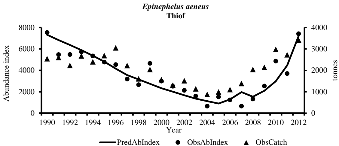
Figure 3.10.4: Epinephelus aeneus . Trends in the observed and estimated abundance indices and diagnostics of the model fit Tendances des indices d'abondance observés et estimés ainsi que des diagnostics du modèle
