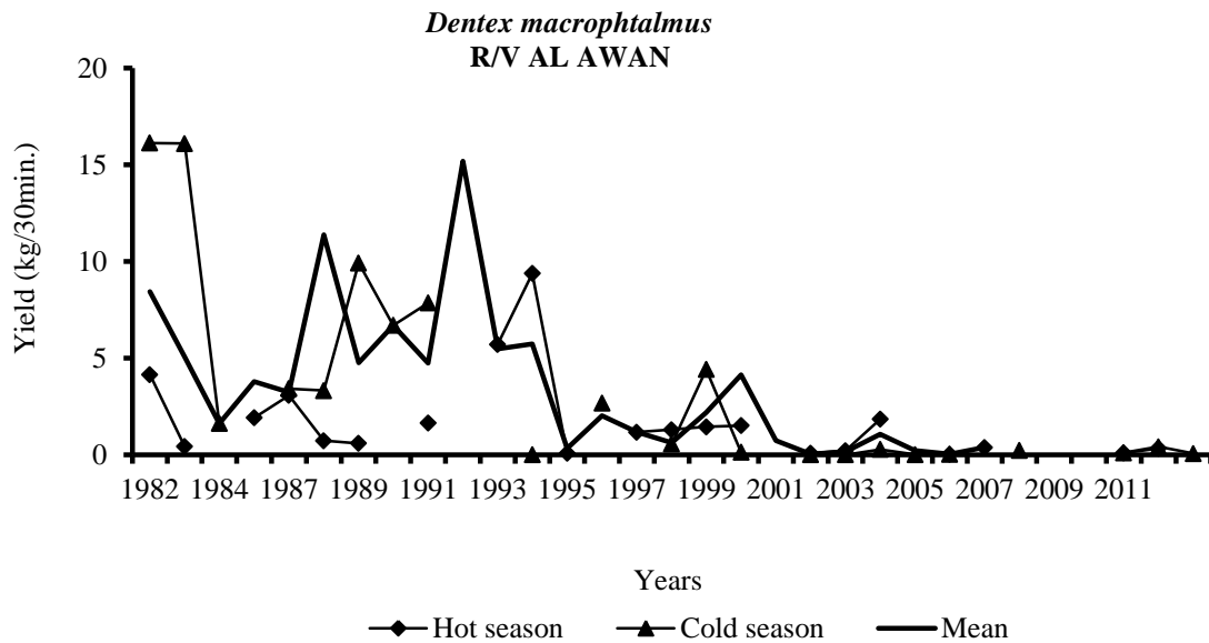
Figure 3.5.3c: Trends in abundance indices (annual average, more than one survey) of Dentex macrophthalmus (kg/30 min) – R/V AL AWAM (Mauritania) Évolution des indices d'abondance (moyenne annuelle, plus d'une campagne par année) de Dentex macrophthalmus (kg/30 min) avec le N/O AL AWAM (Mauritanie)
