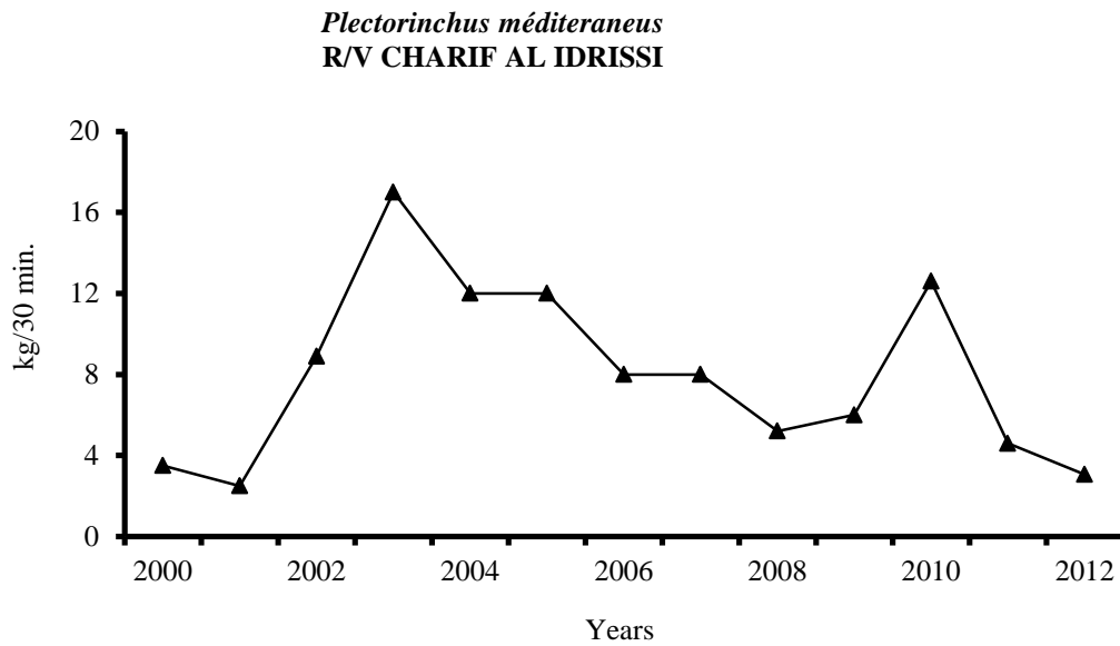
Figure 3.12.3 c . Plectorhinchus mediterraneus . Abundance indices (kg/30 min) obtained during the scientific surveys in Morocco with R/V CHARIF AL IDRISSE Plectorhinchus mediterraneus . Indices d'abondance (kg/30 min) obtenus lors des campagnes scientifiques au Maroc avec le N/R CHARIF AL IDRISSE.
