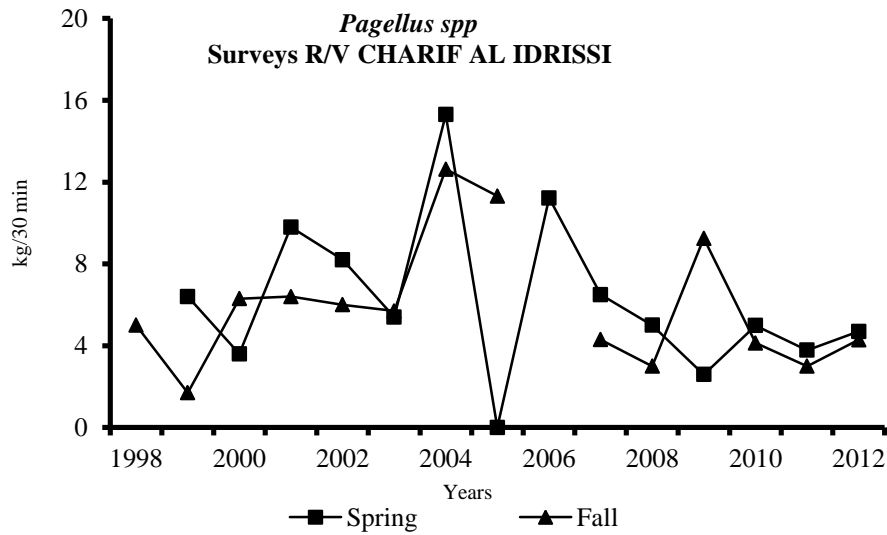
Figure 3.11.3c: Pagellus spp. Abundance indices (kg/30 min) obtained during the scientific surveys in Morocco with R/V CHARIF AL IDRISI/ Pagellus spp. Indices d'abondance (kg/30 min) obtenus lors des campagnes scientifiques au Maroc avec le N/R CHARIF AL IDRISI
