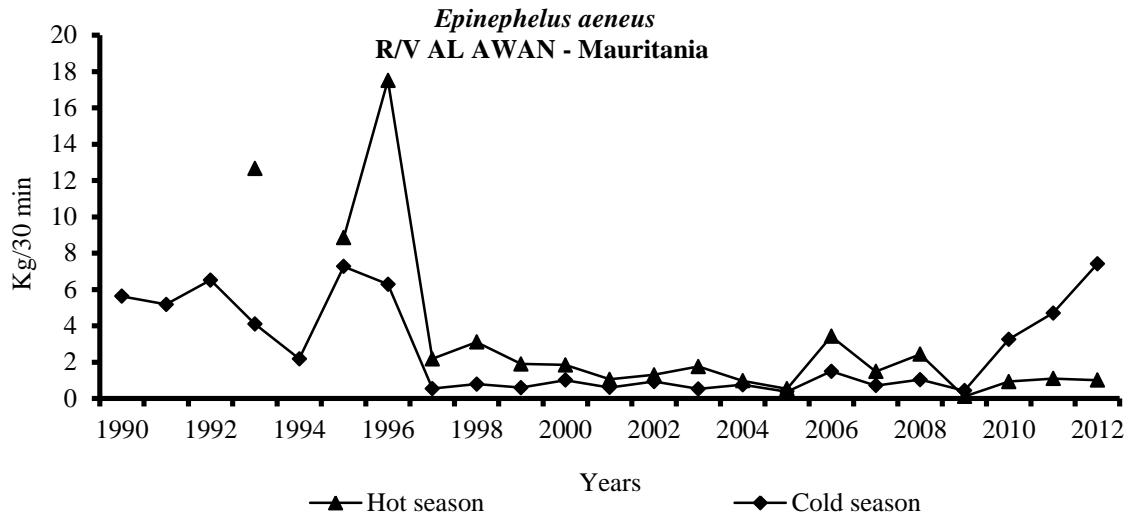
Figure 3.10.3c: Epinephelus aeneus . Abundance indices (kg/30 min) obtained during the scientific surveys in Mauritania with R/V AL AWAM Epinephelus aeneus . Indices d'abondance (kg/30 min) obtenus lors des campagnes scientifiques en Mauritanie avec N/O AL AWAM
