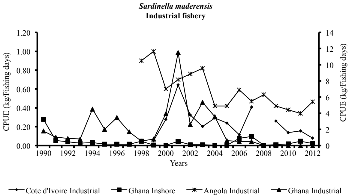
Figure 2.3.1c: CPUE of Sardinella maderensis for industrial fishery/CPUE de Sardinella maderensis pour la pêche industrielle
