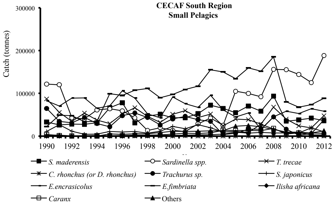
Figure 1.5.1a: Catches of the main species of small pelagics in the southern CECAF region 1990–2008/Captures des principales espèces de petits pélagiques dans la zone sud du COPACE en 1990-2008
