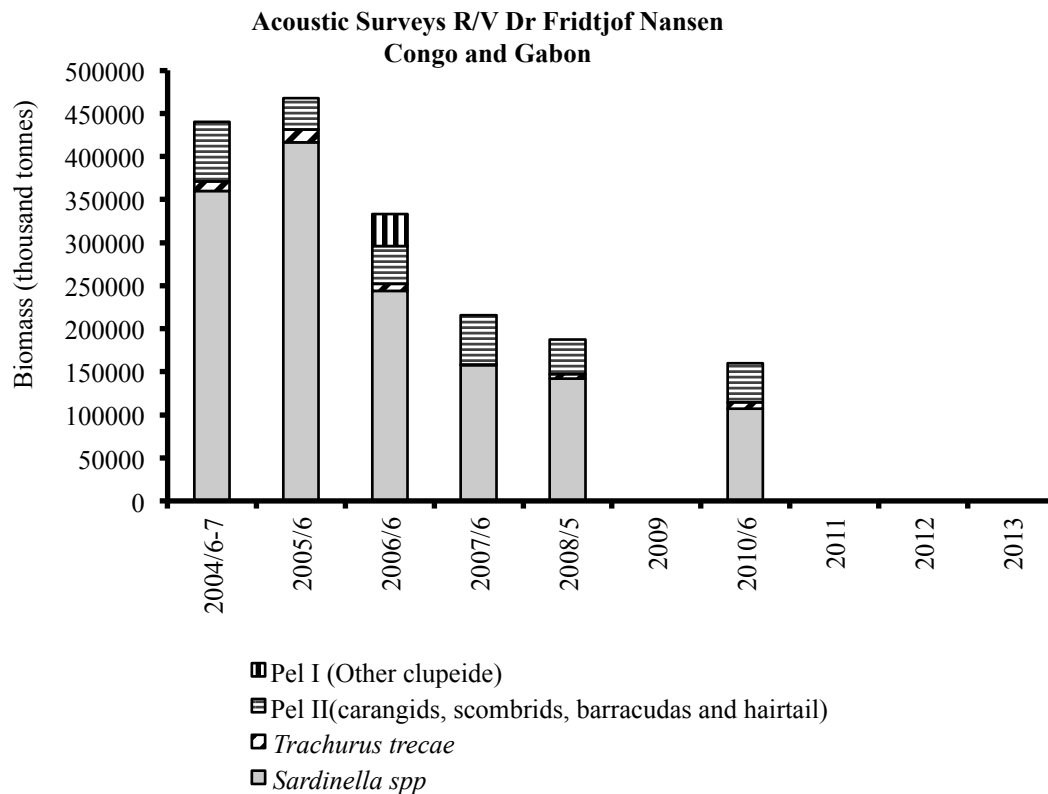
Figure 1.6.1.d: Evolution of biomass (in thousand tonnes) of main pelagic groups estimated by R/V DR. Fridtjof Nansen during the period 2004–2010 (Congo and Gabon)/Evolution de la biomasse (en milliers de tonnes) des principaux groupes pélagiques estimée par le N/R Dr Fridtjof Nansen durant la période 2004-2010 (Congo et Gabon)
