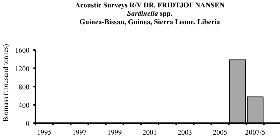
Figure 2.3.2a: Biomass estimates of Sardinella spp. for Northern stock (Guinea-Bissau, Guinea, Sierra Leone and Liberia) for R/V DR. F. NANSEN/Estimations de la biomasse de Sardinella spp. pour le stock nord (Guinée-Bissau, Guinée, Sierra Leone et Libéria) pour le N/R Dr Fridtjof Nansen
