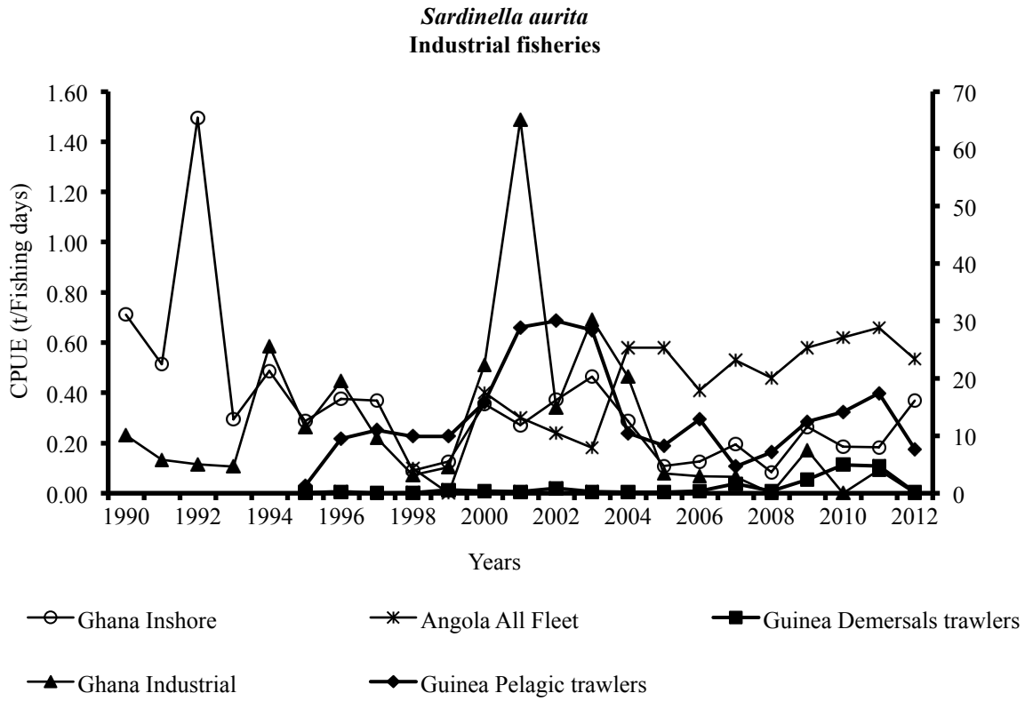
Figure 2.3.1a: CPUE of Sardinella aurita for industrial fishery/CPUE de Sardinella aurita pour la pêche industrielle
