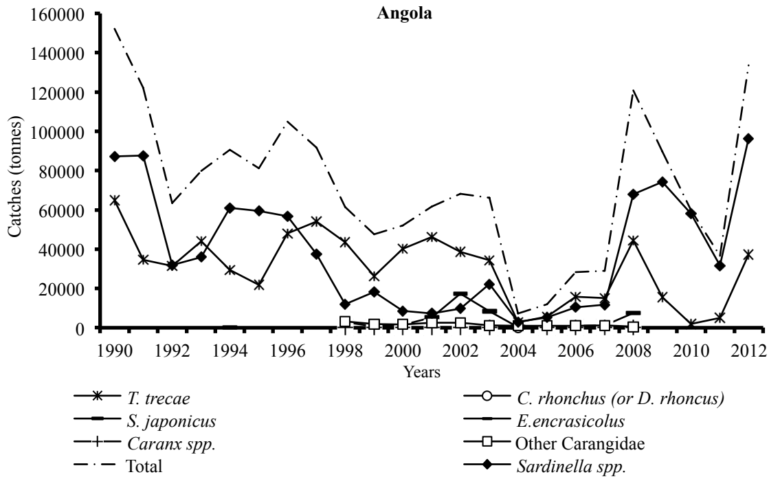
Figure 1.5.1m: Catches of the main species of small pelagics in Angola / Captures des principales espèces de petits pélagiques en Angola
