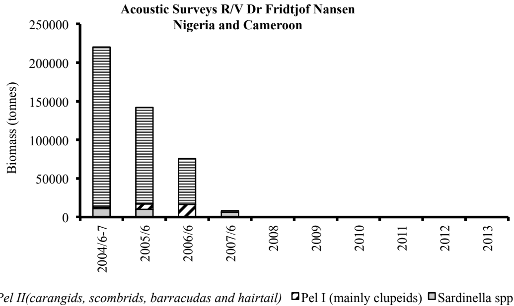
Figure 1.6.1.c: Evolution of biomass (in tonnes) of main pelagic groups estimated by R/V DR. Fridtjof Nansen during the period 2004–2007 (Central Gulf of Guinea: Cameroon and Nigeria)/Evolution de la biomasse (en tonnes) des principaux groupes pélagiques estimée par le N/R Dr Fridtjof Nansen durant la période 2004-2007 (Golfe de Guinée centre: Cameroun et Nigéria)
