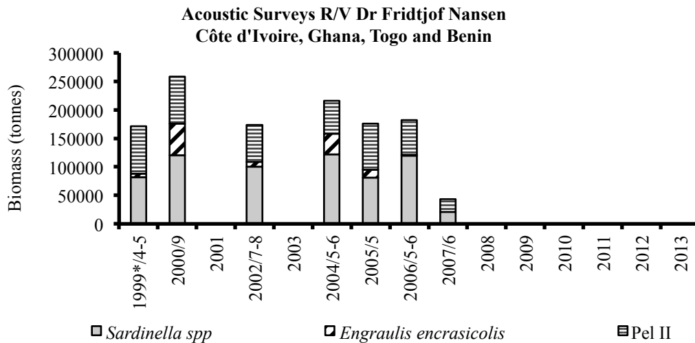
Figure 1.6.1b: Evolution of biomass (in tonnes) of main pelagic groups estimated by R/V DR. Fridtjof Nansen during the period 1999–2007 (Western Gulf of Guinea: Côte d'Ivoire, Ghana, Togo and Benin)/Evolution de la biomasse (en tonnes) des principaux groupes pélagiques estimée par le N/R Dr Fridtjof Nansen durant la période 1999-2007 (Ouest du Golfe de Guinée: Côte d'Ivoire, Ghana, Togo et Bénin)
