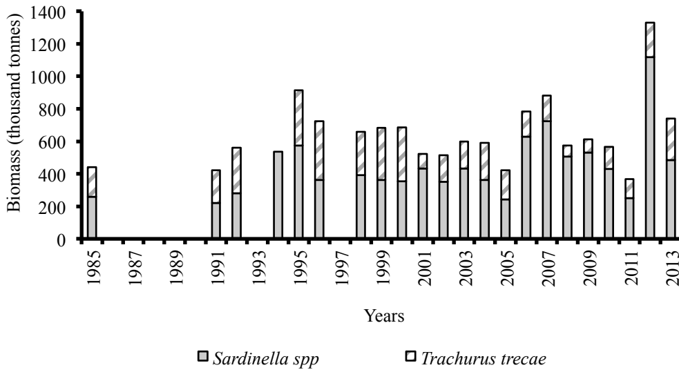
Figure 1.6.1e: Evolution of biomass (in thousand tonnes) of main pelagic groups estimated by R/V DR. Fridtjof Nansen during the period 1985–2013 (Angola)/ Evolution de la biomasse (en milliers de tonnes) des principaux groupes pélagiques estimée par le N/R Dr Fridtjof Nansen durant la période 1985-2013 (Angola)
